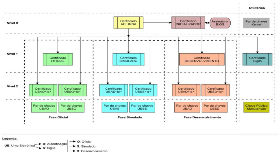
Figura 4.7 – Hierarquia de certificados e chaves da Urna Eletrônica
