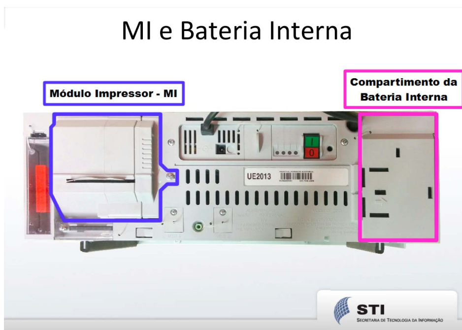
Figura 4.2 – A Urna Eletrônica 2013 – Detalhamento traseiro MI e Bateria Interna.
