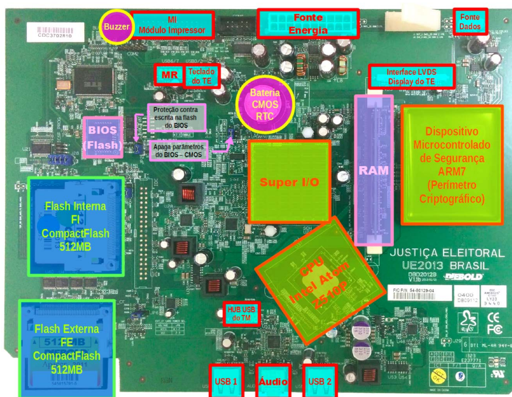
Figura 4.5 – A Urna Eletrônica 2013 – Componentes da placa-mãe.
