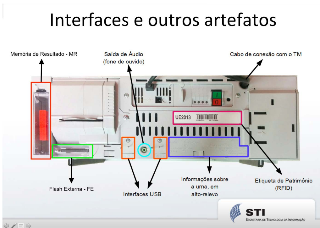
Figura 4.4 – A Urna Eletrônica 2013 – Armazenamento de Dados e Interfaces.
