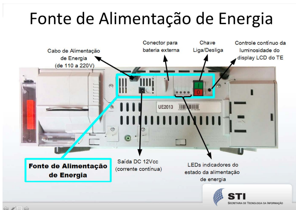
Figura 4.3 – A Urna Eletrônica 2013 – Fonte de Alimentação e Energia.
