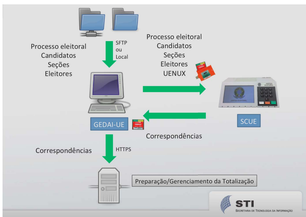
Figura 5.1 – Gerenciador de Dados, Aplicativos e Interface com a Urna Eletrônica
