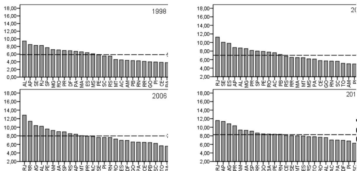
Figura 1. Média do NEP por UF e eleição
