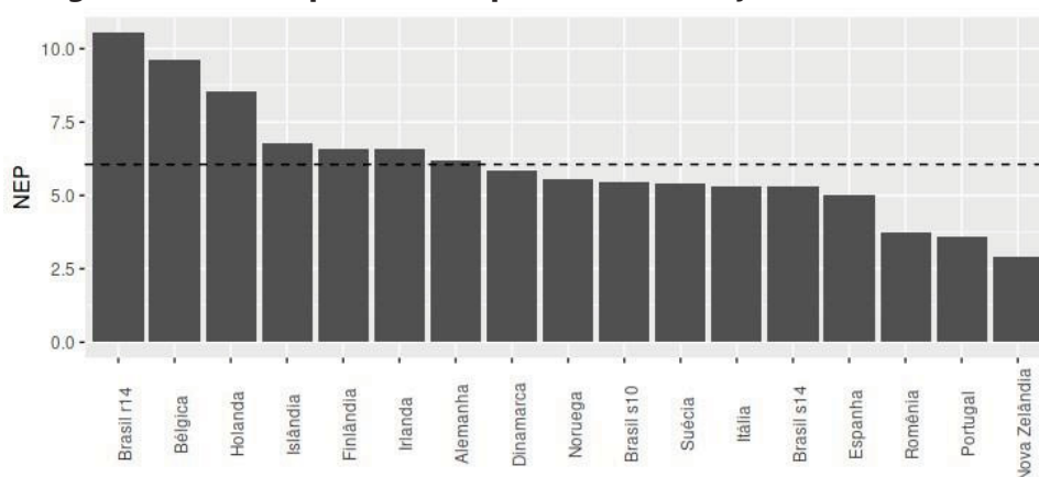
Figura 6. NEP de países multipartidários (eleições mais recentes)
