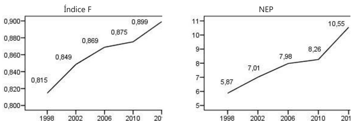
Figura 1. Média da fragmentação partidária nas UF por Eleição
