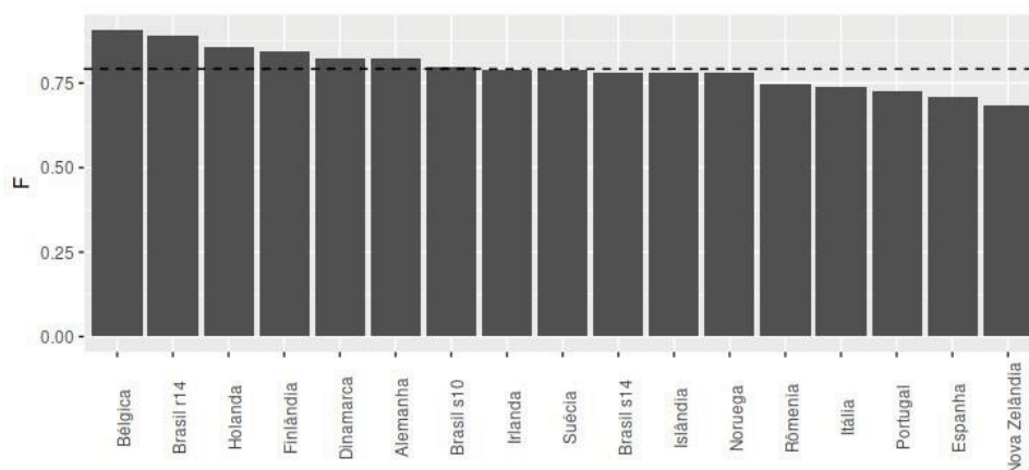
Figura 4. Índice F de países multipartidários 2011
