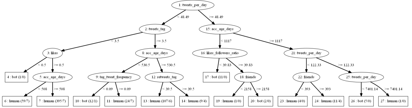
Fig. 4. Modelo de Árvore de Decisão com altura quatro
