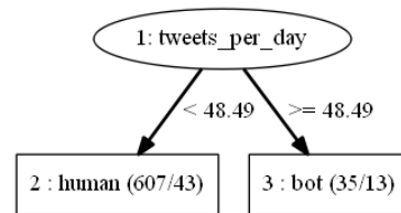
Fig. 1. Modelo de Árvore de Decisão com altura um. Os números entre parênteses representam, respectivamente, o número de usuários classificados nesta categoria e a quantidade destes que está falsamente classificada.
